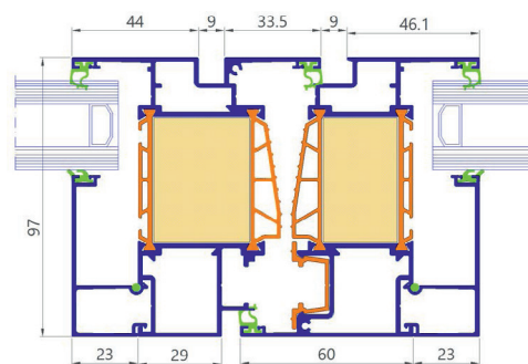
DUBBELE VLEUGEL HORIZONTALE DOORSNEDE
