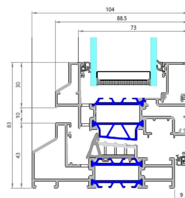
Doorsnede Steellook (*)
