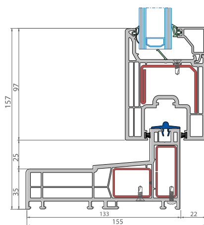
Verticale snede
