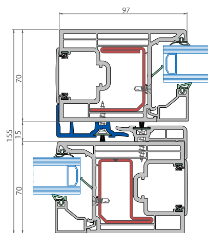
Horizontale snede
